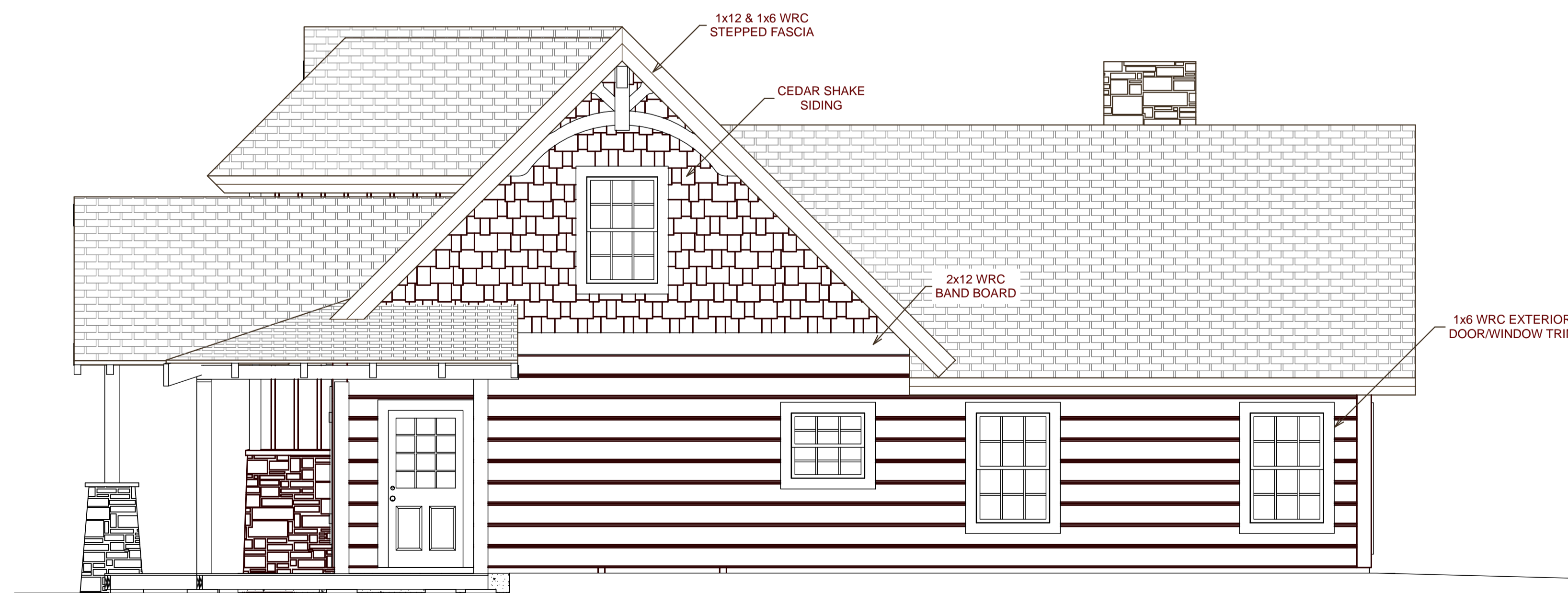
RIGHT ELEVATION
